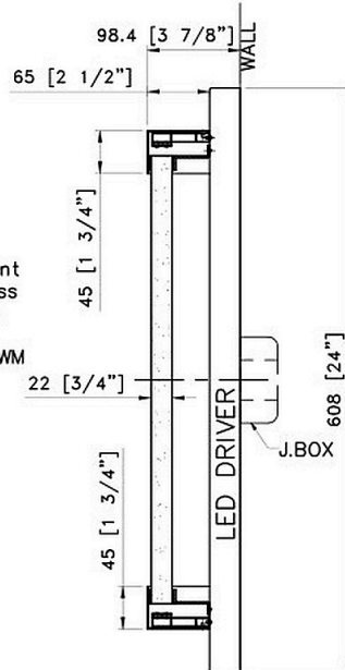
SIDE VIEW SCALE: 1:5
