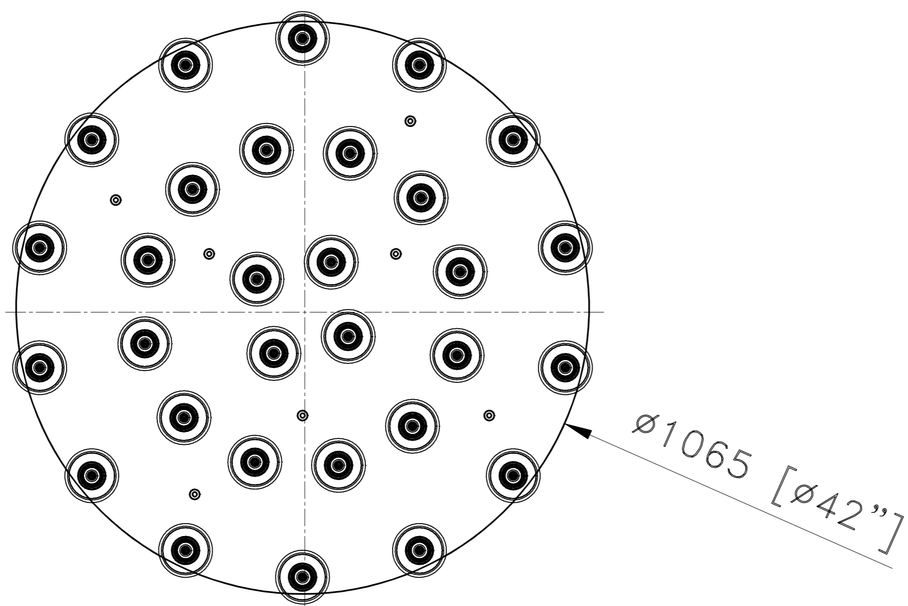
BOTTOM VIEW SCALE: 1 : 20
