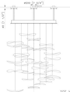
SIDE VIEW SCALE: 1: 30
