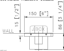
TOP VIEW SCALE: 1 : 5
