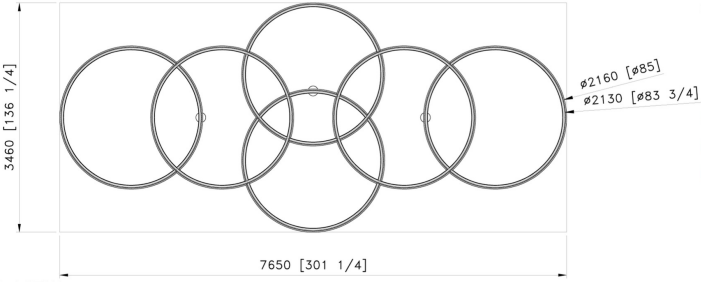
BOTTOM VIEW SCALE: 1 : 50
