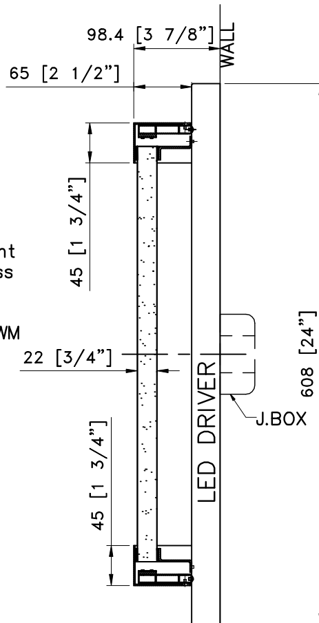
SIDE VIEW SCALE: 1:5
