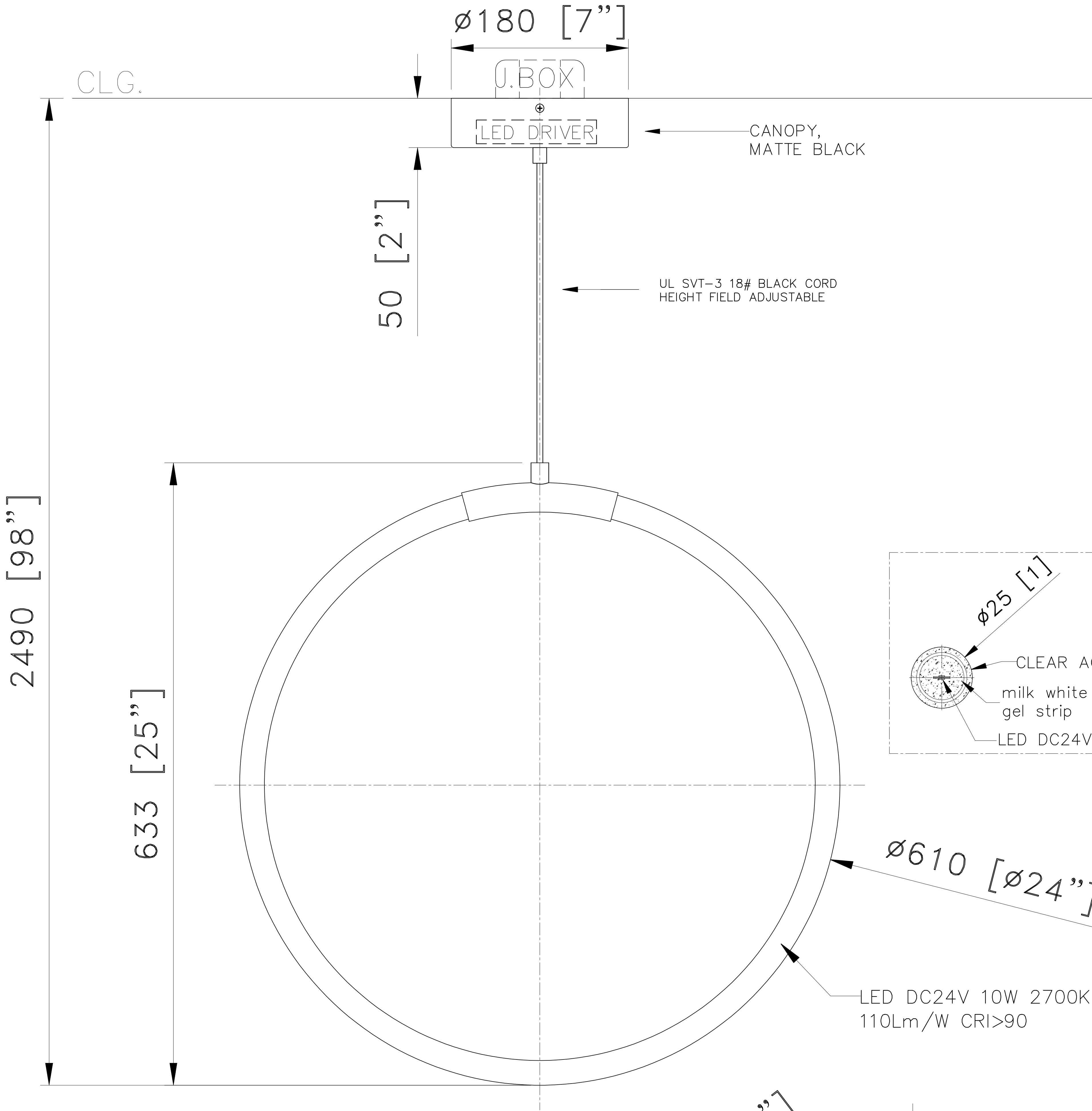
FRONT VIEW SCALE: 1 : 9
