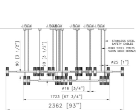
SIDE VIEW SCALE: 1 : 40
