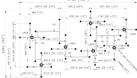
TOP VIEW SCALE: 1 : 40
